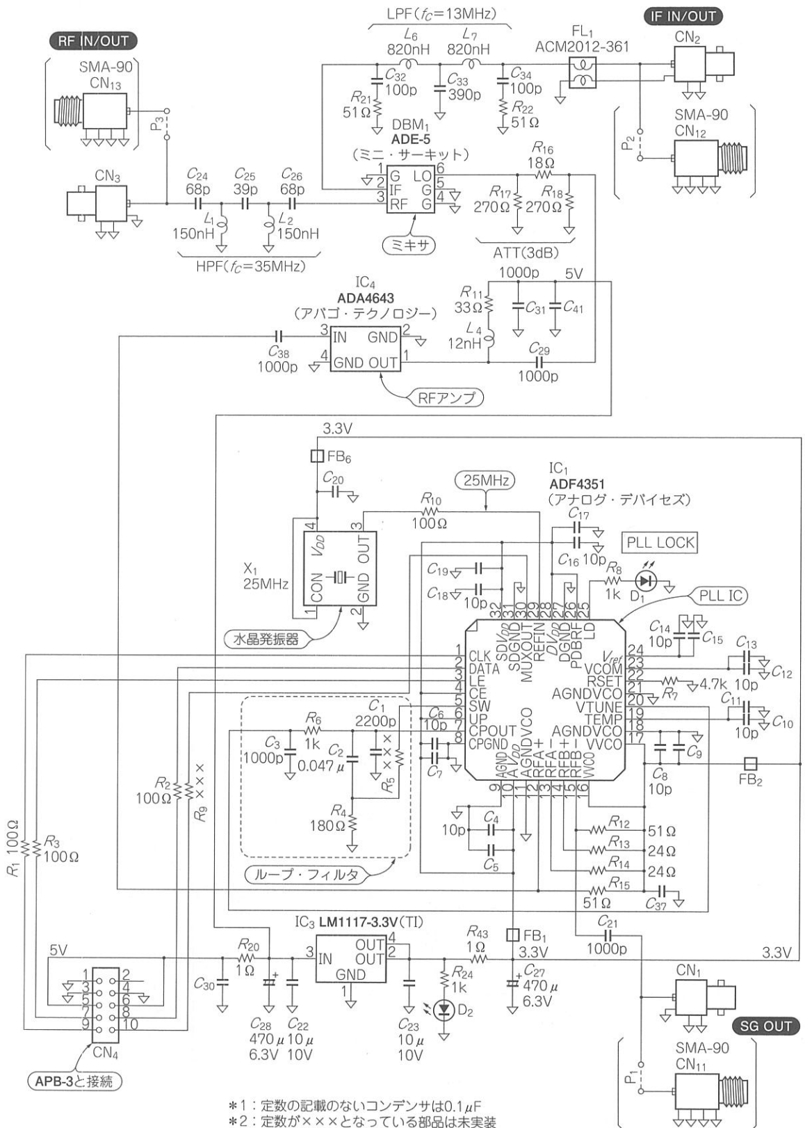
図3 1 GHz RFフロントエンド・アダプタ SAE-1の回路
